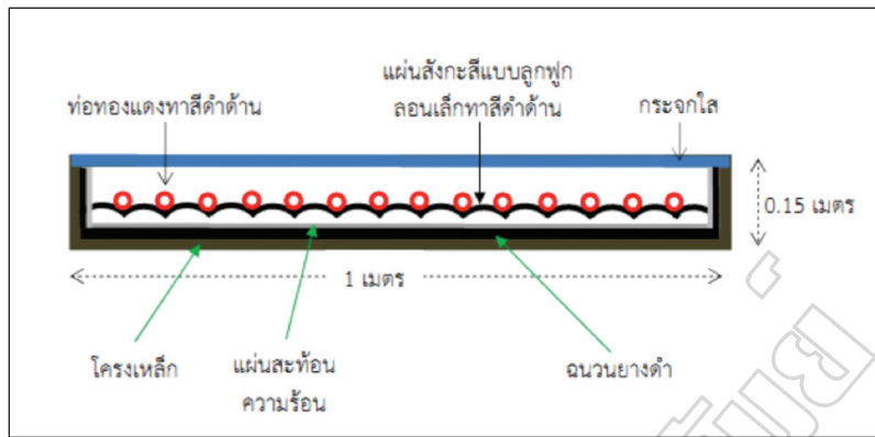
ภาพที่ 2 ภาคตัดขวางโครงสร้างและส่วนประกอบของตัวเก็บรังสีอาทิตย์
