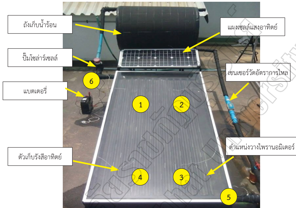
ภาพที่ 5 การติดตั้งเครื่องมือวัด
